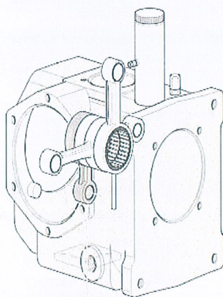
KOT Cilindro 4° stadio SOL-300R
