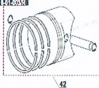
KIT Pistone 1° stadio 8.41.001/R
