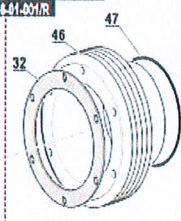
KIT Cilindro 1° stadio 8.41.001/R
