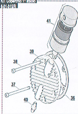
KIT Copertura 1° stadio 8.41.001/R
