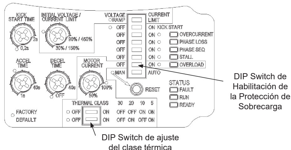
Figura 4.10 - Habilitación e ajuste del protección de sobrecarga
