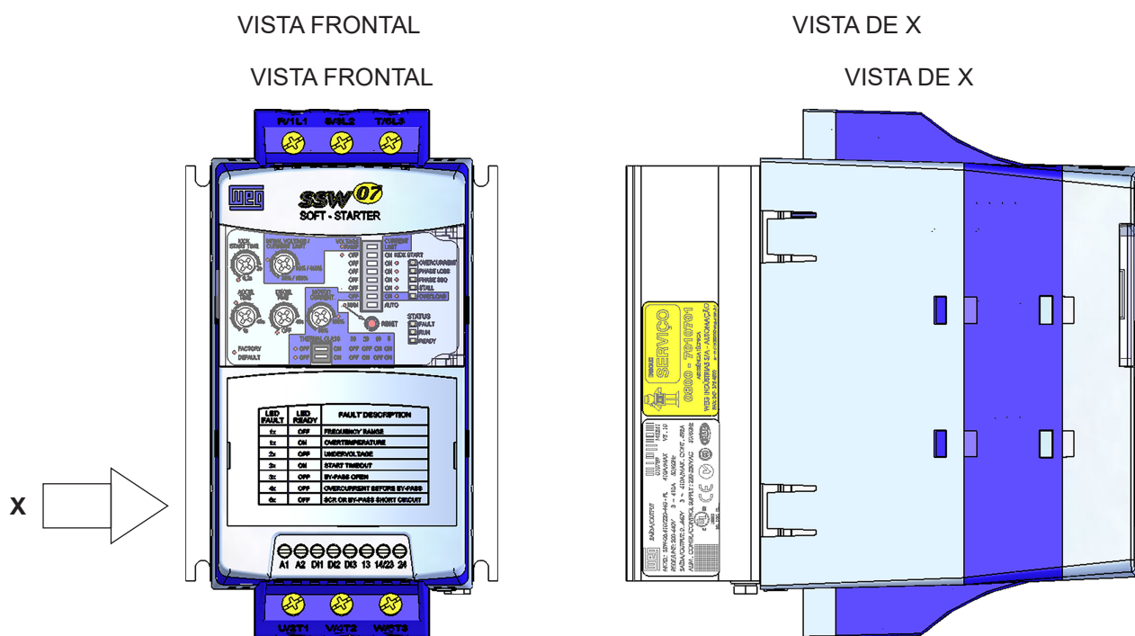
Figura 2.4 - Localização das etiquetas da Soft-Starter SSW-07
